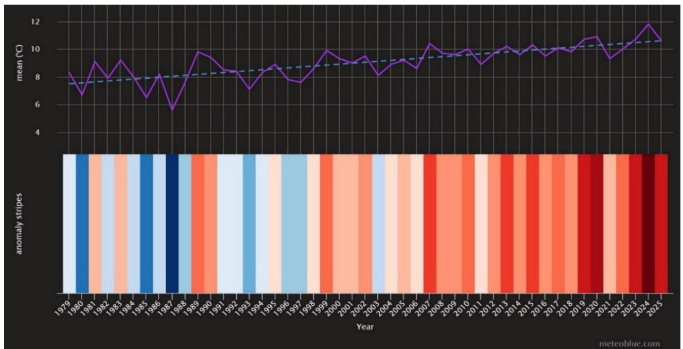
Рисунок 2.2 Річна зміна температури
