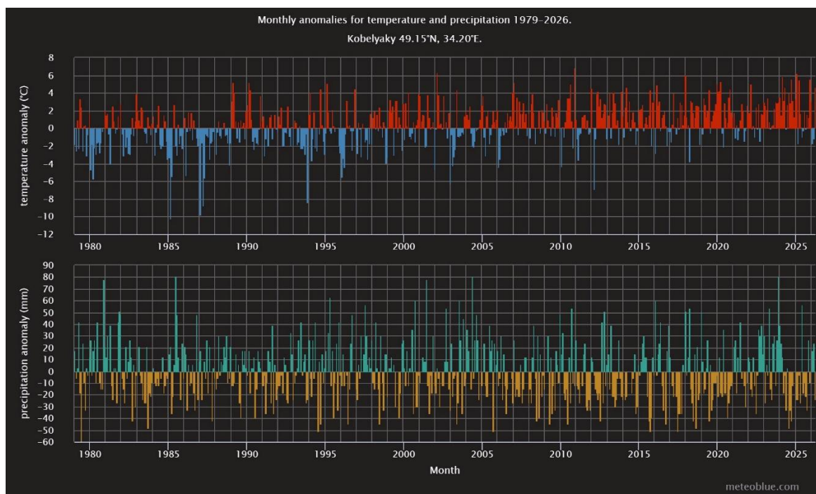
Рисунок 2.4 Місячні аномалії температури й опадів – зміна клімату
