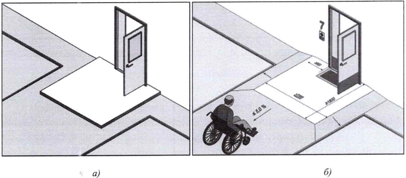
Рисунок 1.3. Облаштування доступного безбар'єрного входу в будинок в разі 1 або 2 сходинок танку: а – наявний стан; б) – організація похилої площини входу
