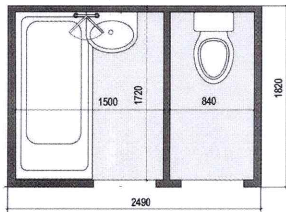
Рисунок 3.20. Приклад типового санітарно- гігієнічного приміщення. Тип 1
