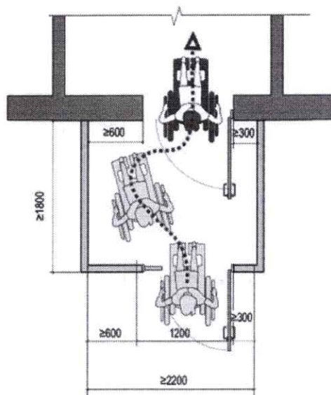
Рисунок 1.35. Схема маневрування в межах тамбура
