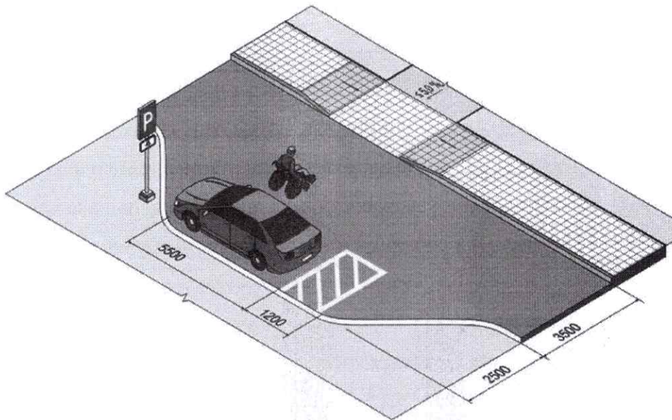
Рисунок 1.1. Місця для паркування автомобілей людей з інвалідністю
