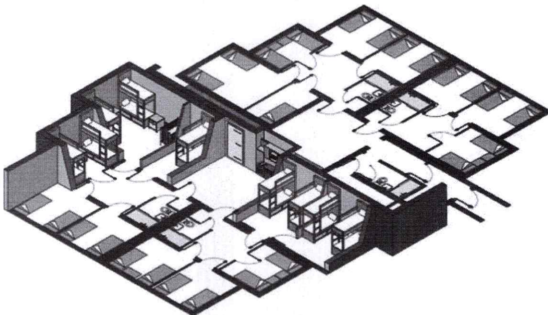
Рисунок 2.7. Схема облаштування укриття в будинку з приватними коморами
