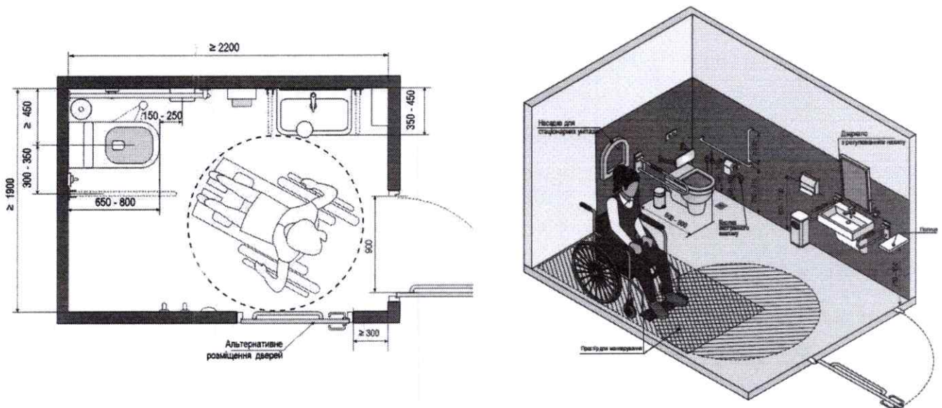
Рисунок 2.5. Схема обладнання інклюзивного санітарно-гігієнічного приміщення
