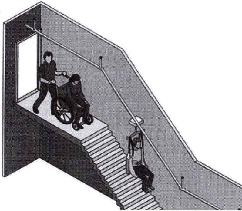
Рисунок 2.2. Схема влаштування стельового підіймального пристрою
