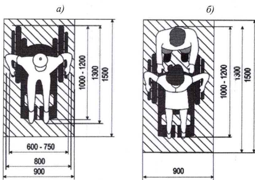
Рисунок 3.2. Габарити людини на кріслі колісному: а – при самостійному користуванні; б – за допомогою помічника
