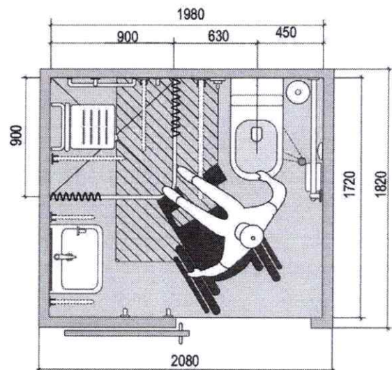
Рисунок 3.21. Приклад типового санітарно- гігієнічного приміщення. Тип 2
