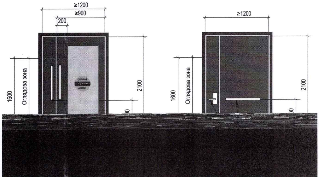
Рисунок 1.10. Двері оглядовими панелями
