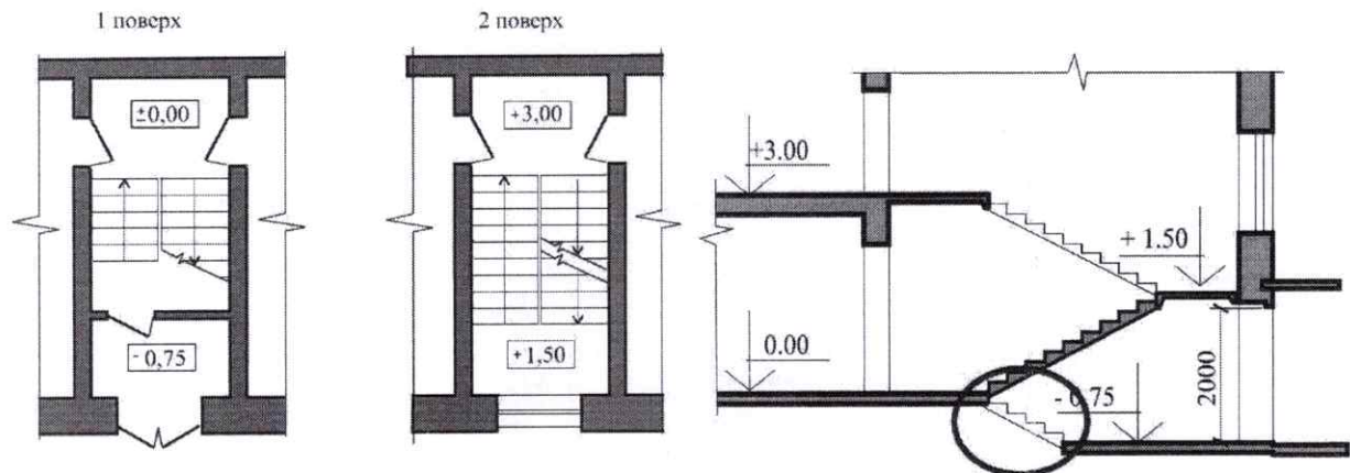
Рисунок 1.36. Сходинок цокольного поверху типове рішення
