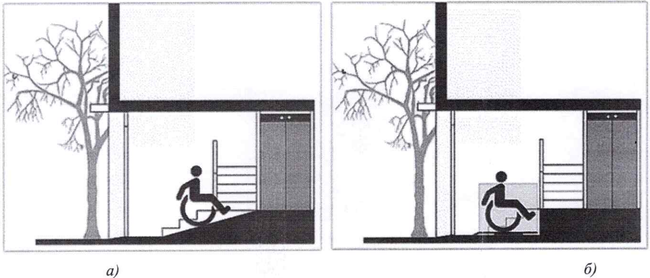
Рисунок 1.12. Методи забезпечення доступності до ганку:
