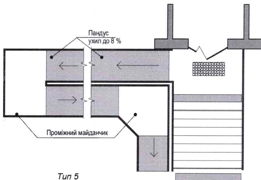
Рисунок 1.23.3. Типи облаштування вхідної групи (продовження): д) П-подібний пандус
