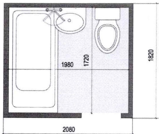
Рисунок 3.22. Приклад типового санітарно- гігієнічного приміщення. Тип 3
