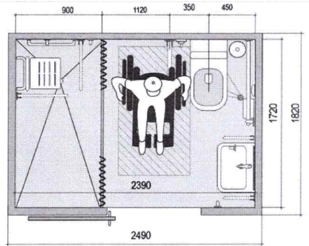
Рисунок 3.20. Приклад типового санітарно- гігієнічного приміщення. Тип 1
