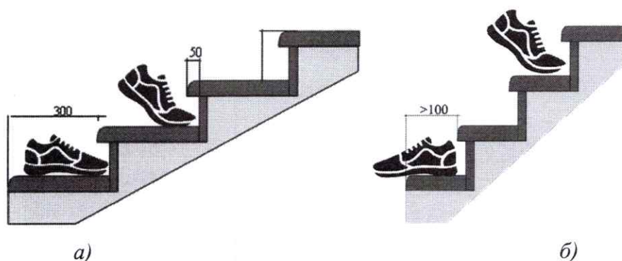
Рисунок 1.13. Безпека на сходах:
