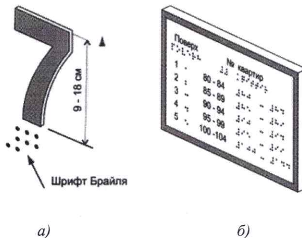
Рисунок 1.6. Інформаційні таблиці: а – номер під'їзду; б – номери квартир
