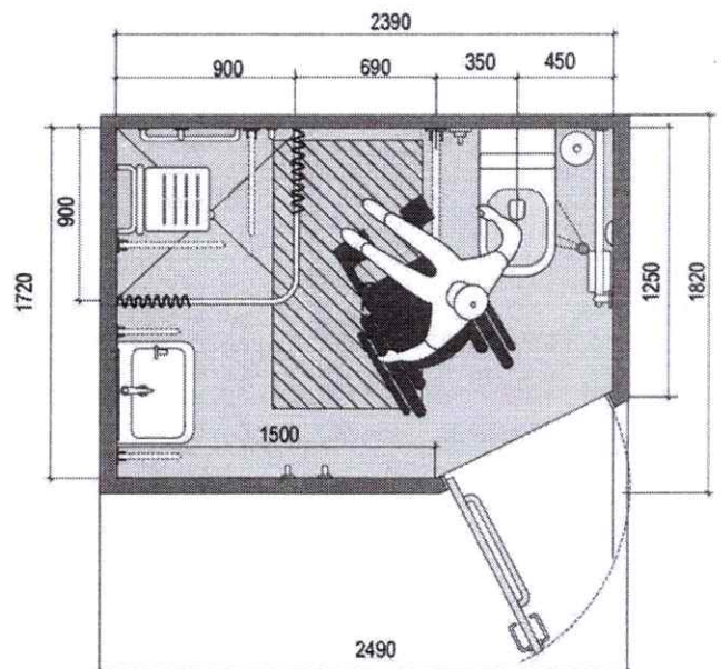
Рисунок 3.21. Приклад типового санітарно- гігієнічного приміщення. Тип 2
