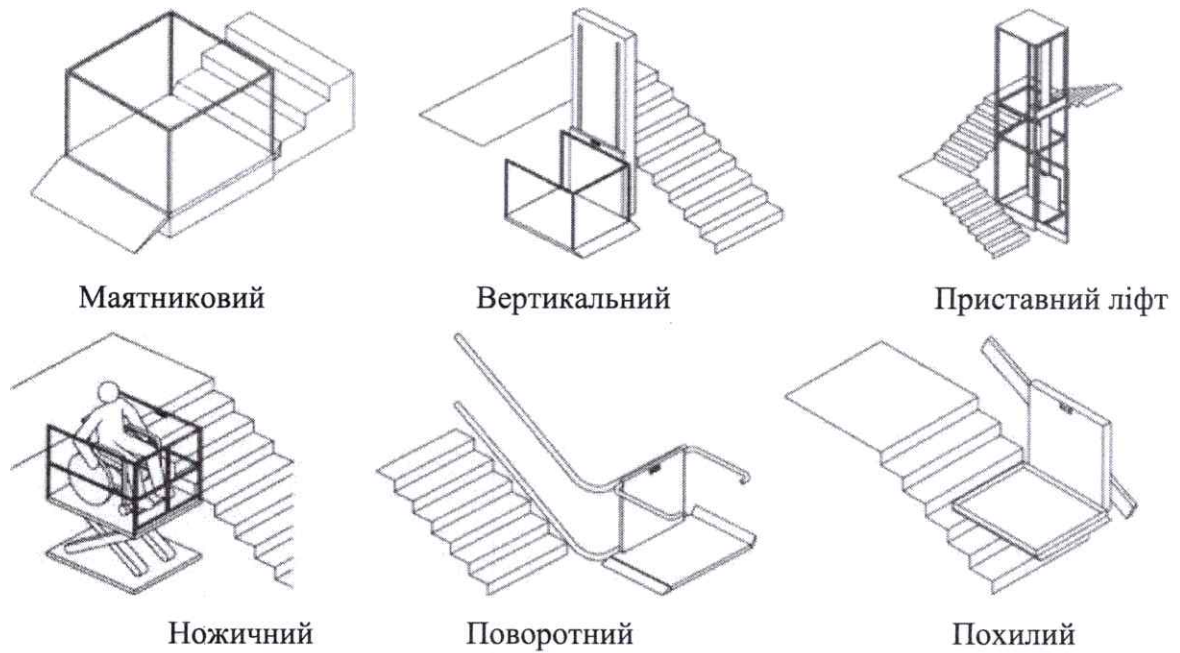
Рисунок 1.41. Типи підіймальних пристроїв
