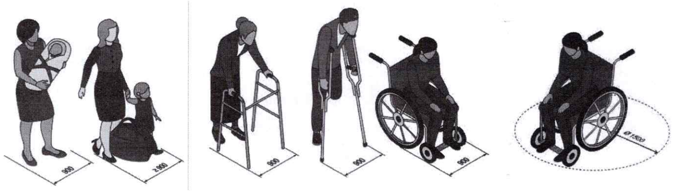
Рисунок 1.5. Простір руху необхідний для маломобільної групи населення
