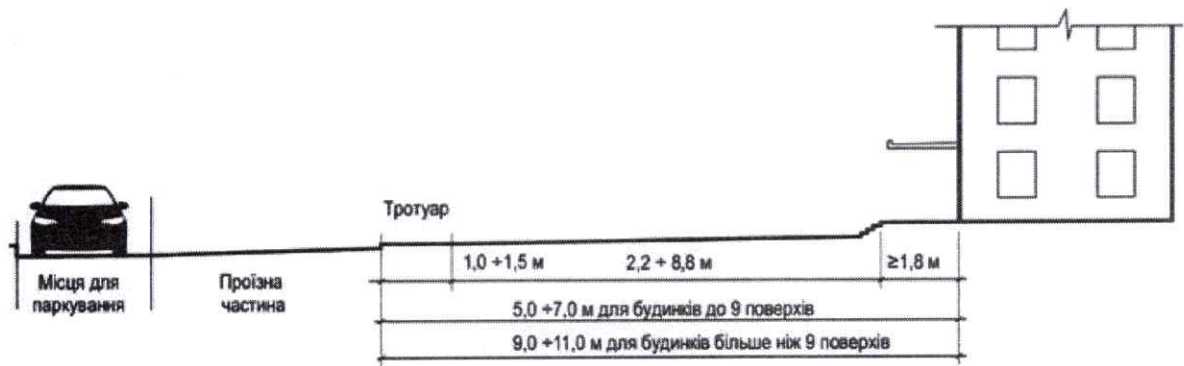
Рисунок 1.2. Нормативна відстань від стін будинків до пожежного проїзду
