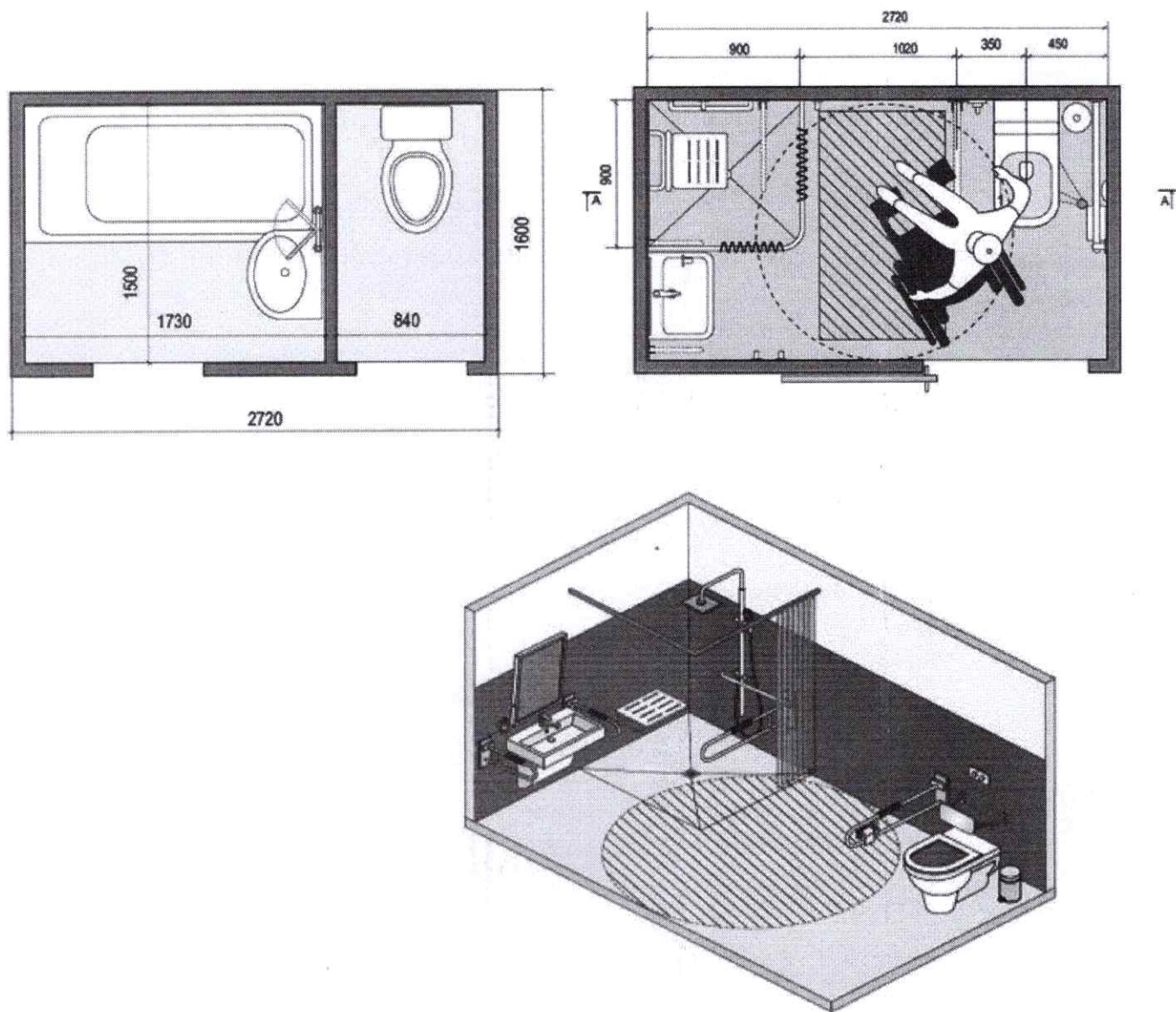
Рисунок 3.23. Приклад типового санітарно-гігієнічного приміщення. Тип 4
