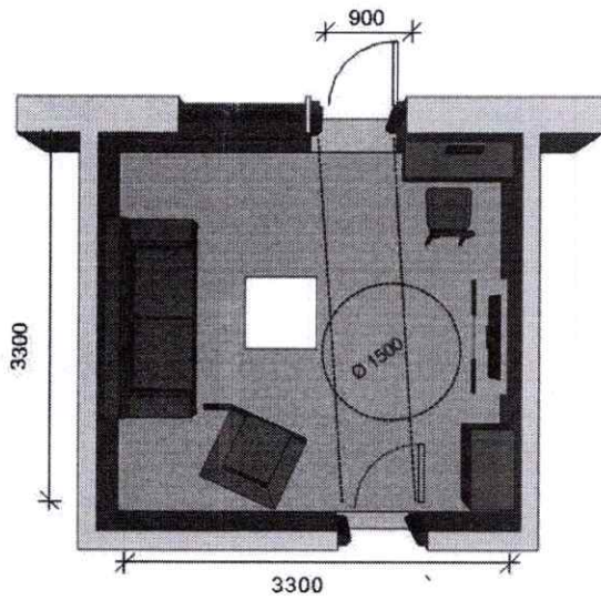
Рисунок 3.8 Схема умеблювання доступної вітальні
