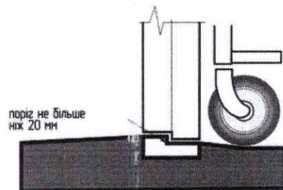
Рисунок 1.9. Порог вхідного вузла
