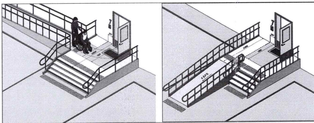
Рисунок 1.25. Варіанти влаштування пандуса для ганків висотою до 75 см: а – вздовж стіни будинку; б – прямий пандус у напрямку тротуару.
