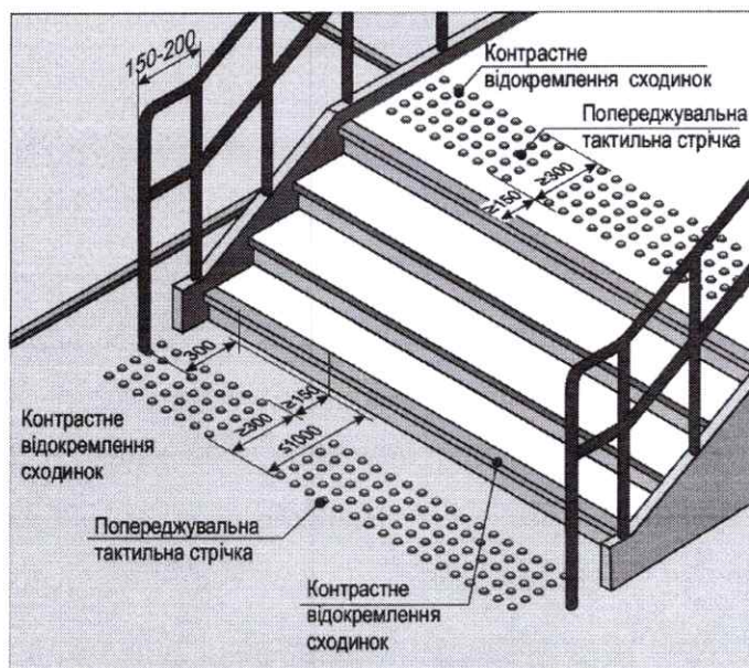
Рисунок 1.14. Облаштування сходинок
