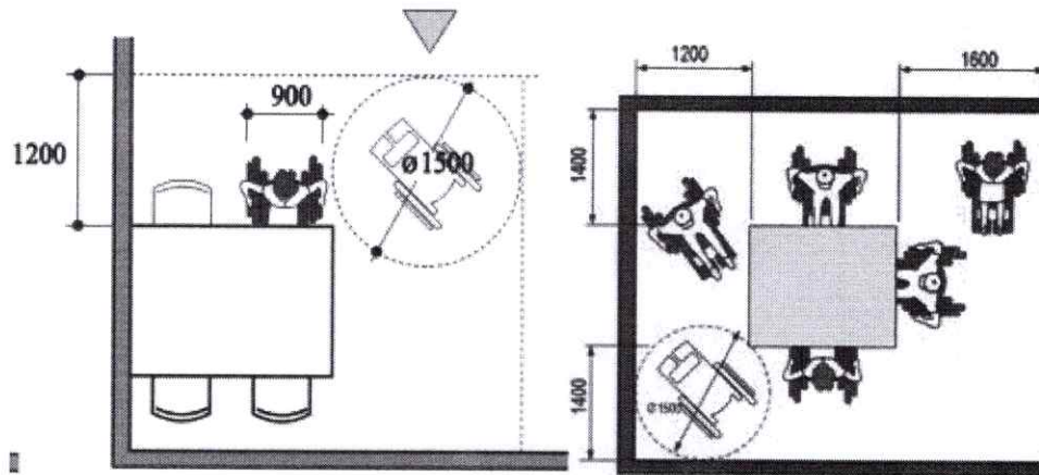
Рисунок 3.10. Нормативні відстані в їдальні
