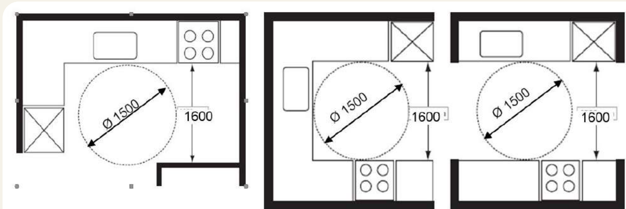
Рисунок 3.14. Варіанти розміщення обладнання в робочій кухні
