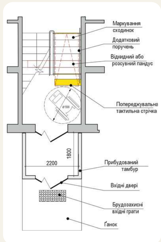
Рисунок 1.38. Схема адаптації входів до першого поверху в будинках типових серій
