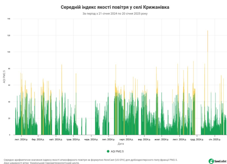
Рис. 3. Динаміка Індексу якості повітря у Фонтанській громаді (за даними Saveecobot)
