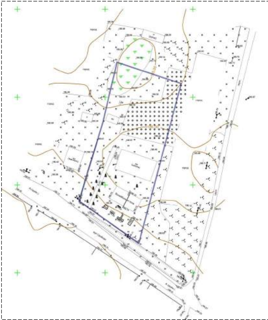
Рис. 1.3. Розташування ділянки на топографо-геодезичній зйомці
